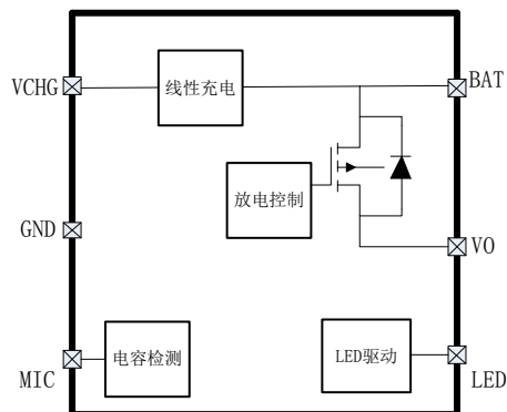
图 3 系统框图
