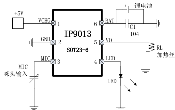
图 4 典型应用原理图
